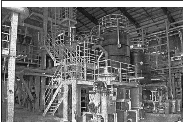
廃石膏結晶大型化処理プラント
